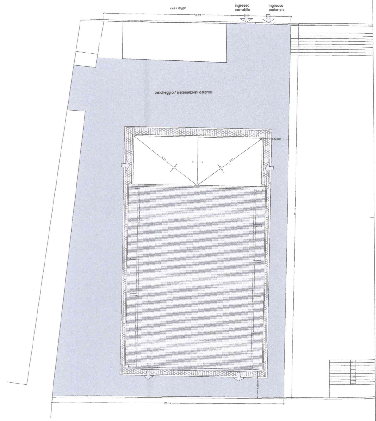
planimetria generale - scala 1:200
